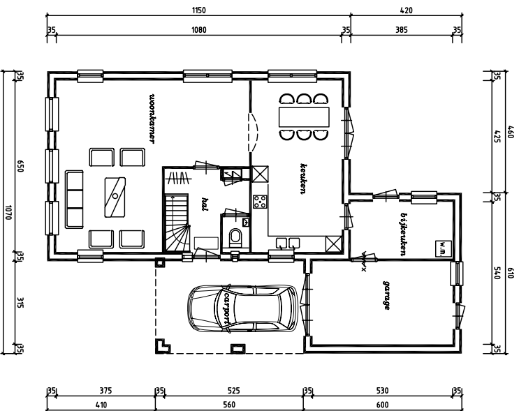
Begane grond
